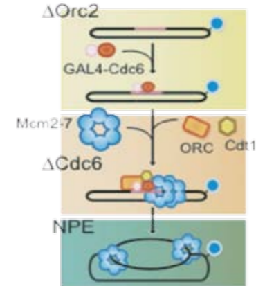
図2: 特定のDNA配列上にpre-RCを形成させる。
