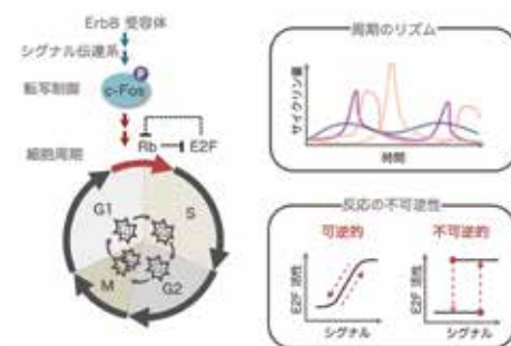
図1. ErbB受容体シグナル伝達による細胞周期制御
