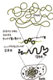
図1 DNAはヒストンなどのタンパク質やRNAとともにクロマチンを形成し核の中に納められている
