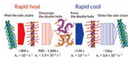
図1. 急加熱、急冷に伴うゼンサン分子のコンホメーション変化の模式図とその時定数
