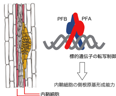
図1. 内鞘細胞の持つ側根形成能はPFA/PFB転写因子複合体に支配されている。内鞘(左図、赤色)は自発的なオーキシニンピークの形成、オーキシニンに応答した不等分裂と側根原基の組織化能を持っています。私たちは、内鞘細胞が持つこの特有の能力は転写因子複合体PFA/PFBによって作られていることを見出しました。
