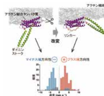
図1. タンパク質エンジニアリングで逆方向性の分子モーターを創る(Furuta et al., Nat Nanotech 2017)。
