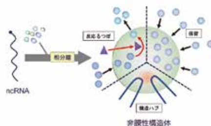
図3. ncRNAによる非膜性構造体の構築機能。ncRNAが一群の天然変性タンパク質を集約して相分離を誘発し非膜性構造体を形成する。形成された構造体の働きとして、反応する、係留、構造ハブの3つの制御機能が提唱されている。
